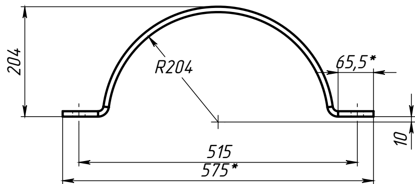
Поз.4 (Полухомут)
