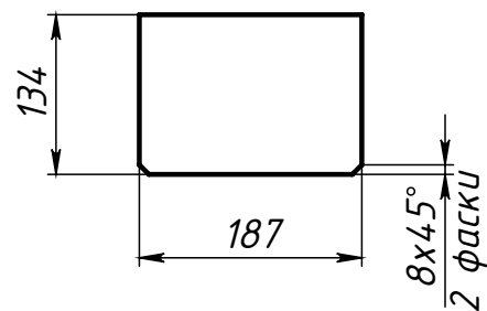
Поз.6 (Ребро)
